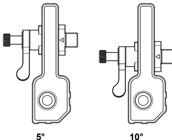
Unterer Männlicher Bügel
