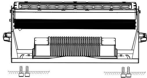
Oberflächenmontage
