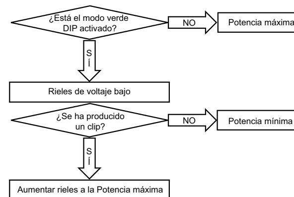
Figura 9.2.1 Cómo funcionan los interruptores DIP Green Power
