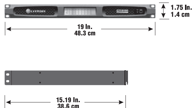
Figura 4.2.1 Dimensiones de la serie CT
