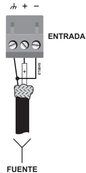
LÍNEA DESEQUILIBRADA
