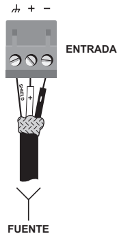
LÍNEA EQUILIBRADA
