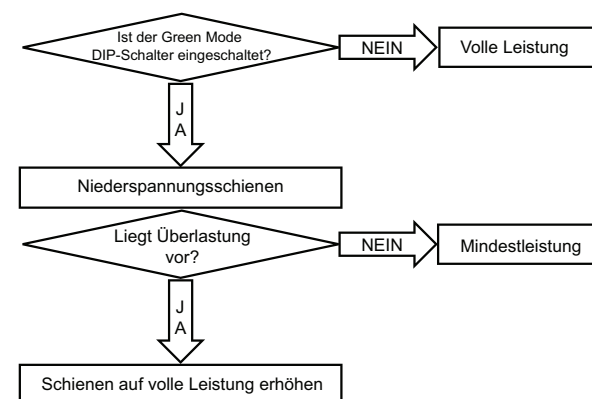
Abb. 9.2.1 Funktion der Green Power DIP-Schalter
