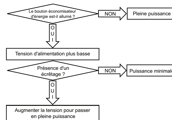
Schéma 9.2.1 Fonctionnement du commutateur DIP économisateur d'énergie
